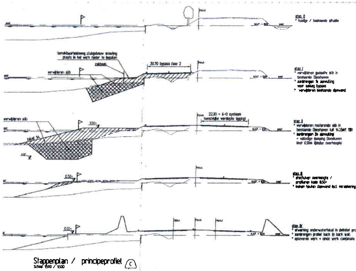
Tekening Dwarsprofiel
